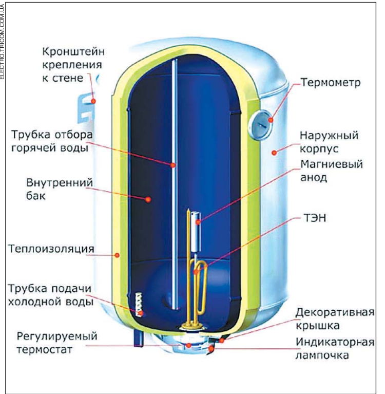
Водонагреватель изнутри
